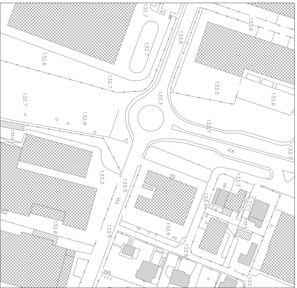
STRALCIO AEROFOTOGRAMMETRICO
